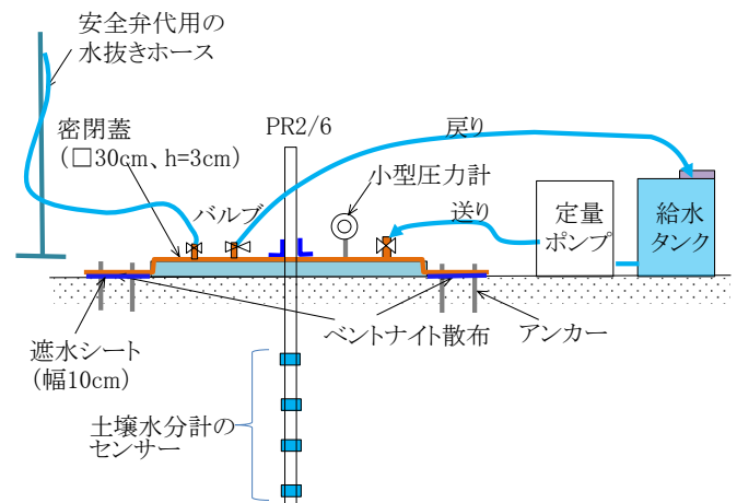
原位置不飽和測定装置の概要
