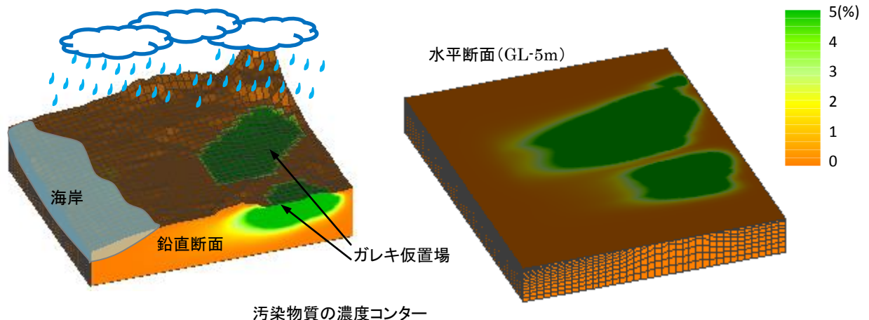
汚染物質の濃度コンター
