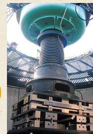
灯台レンズ用免震装置
