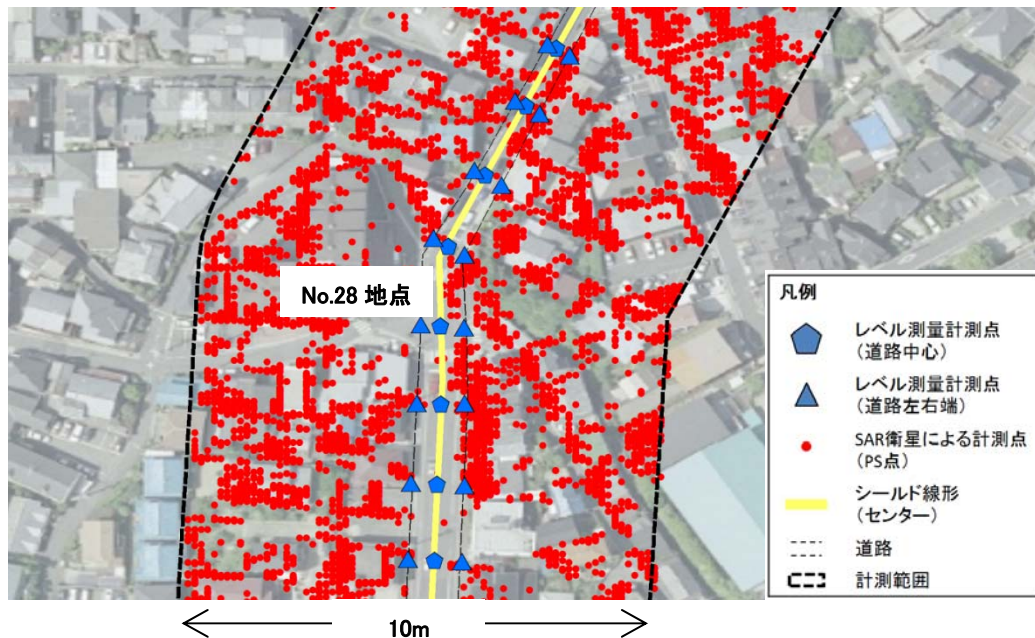
図-3 No.28 地点付近における計測点の比較
