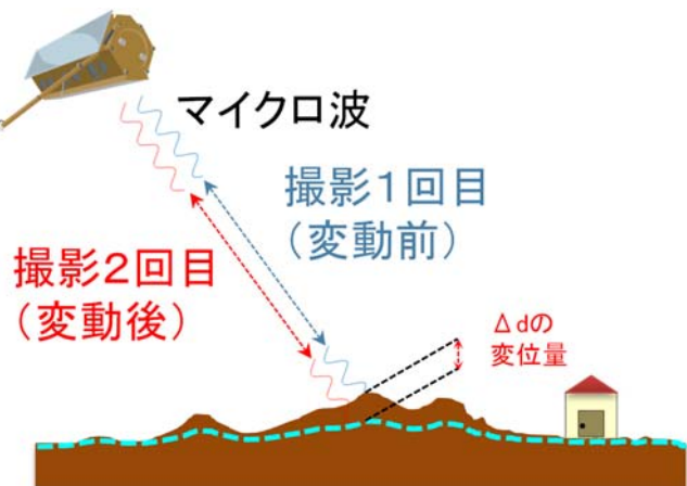
図-1 SAR 衛星による地表面変位測量の概念
