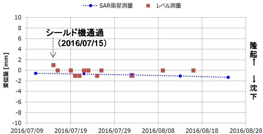
図-2 No.28 地点付近における変位測量結果の比較
