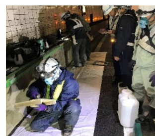
作業時入力(断面修復工)
